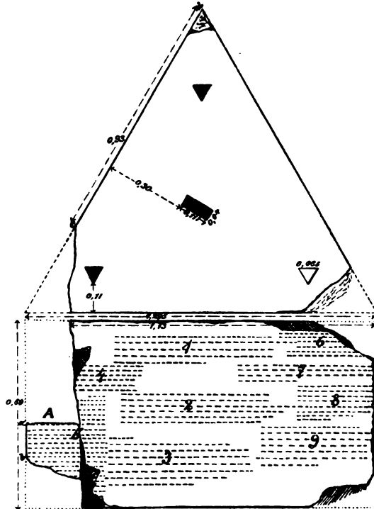
fig. II (1 : 20).
